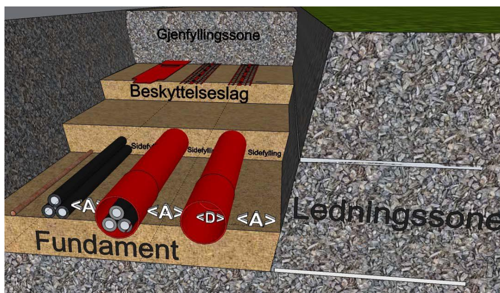
Figur 1 Grøftbeskrivelse- kabelrørlegget
