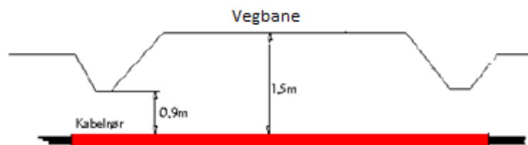
Figur 6 Dybde under veg ved kryssing
