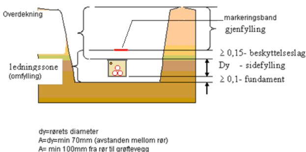
Figur 7 Kabelaer lagt i betongkanal.
