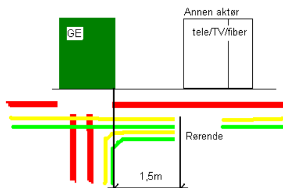
Figur 10 Røravslutning av annen aktør ved Vevigs kabelfordelingsskap
